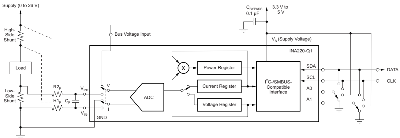
通用负载、低侧或高侧感测
