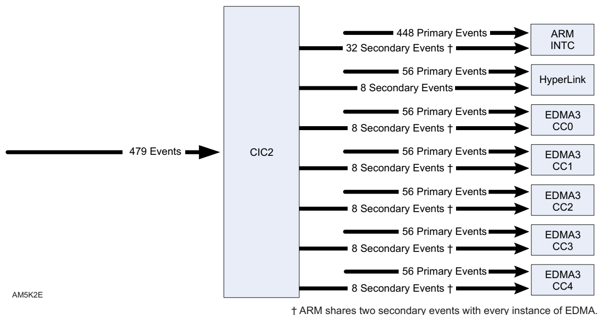
图 6-4. Interrupt Topology
