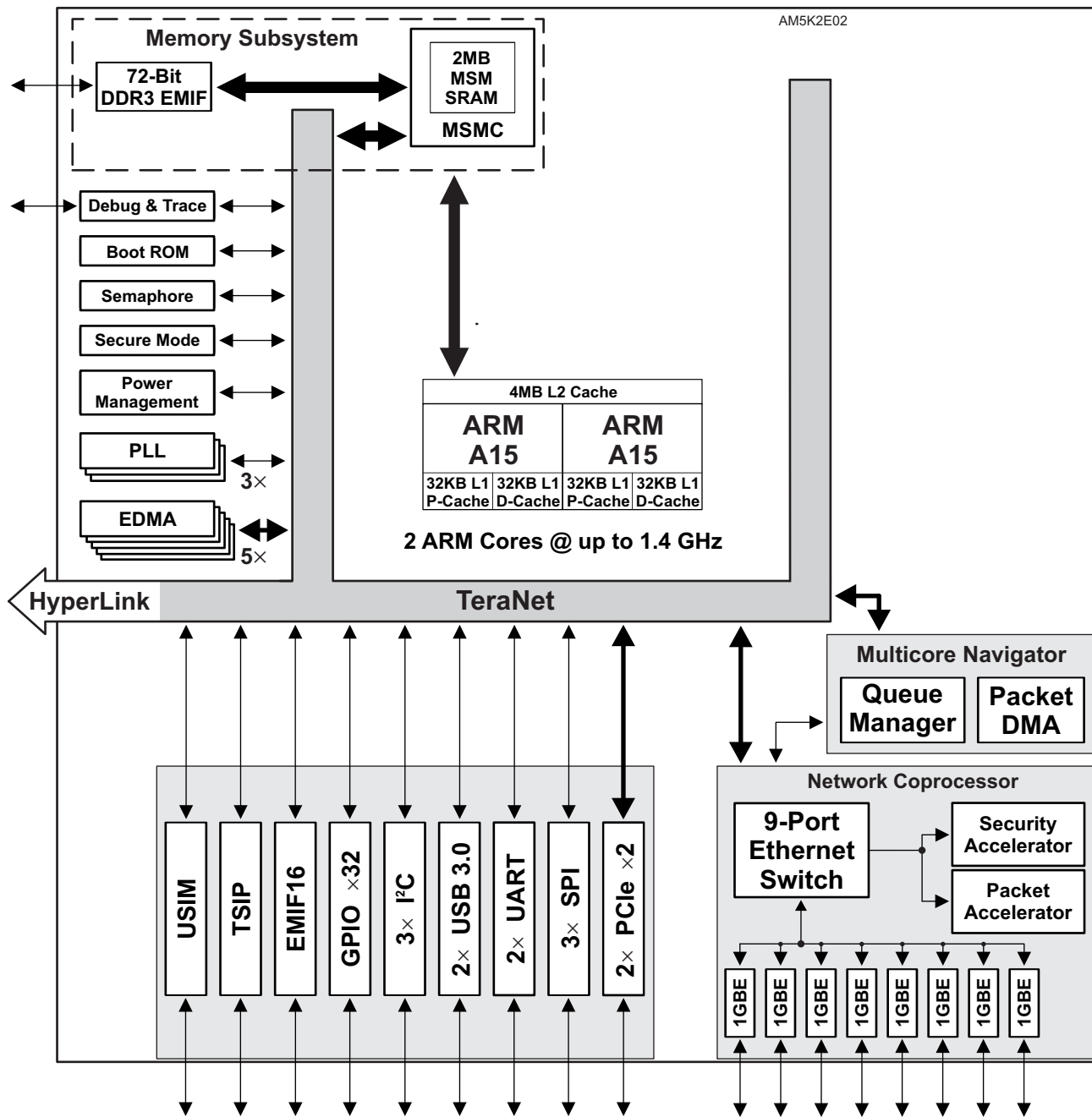
图 1-2. AM5K2E02 功能框图
