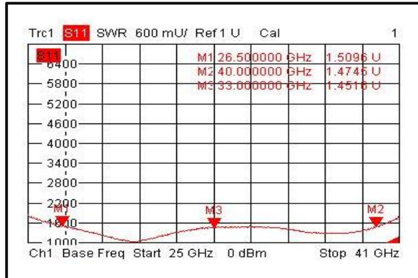
VSWR 1
