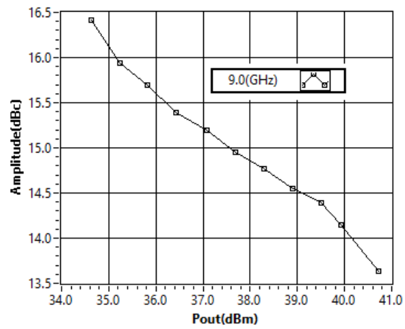
IM3 Test (dBc) vs. Pout (dBm)
