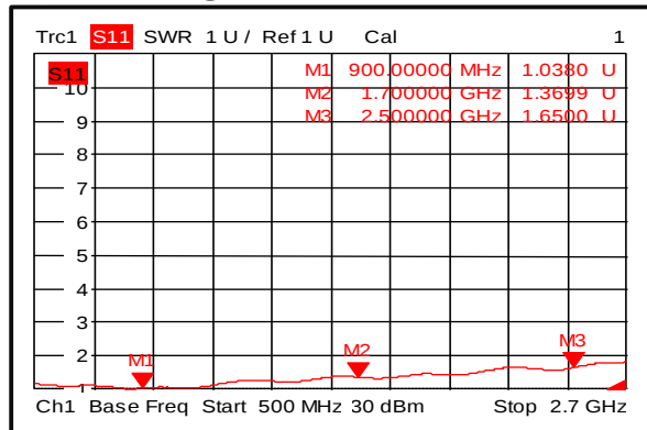
Input VSWR@-45°C
