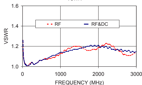
ZFBT-33-75-FT+ VSWR
