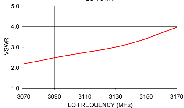
MCA-36FLH+ LO VSWR
