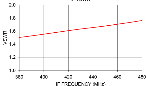
MCA-36FLH+ IF VSWR
