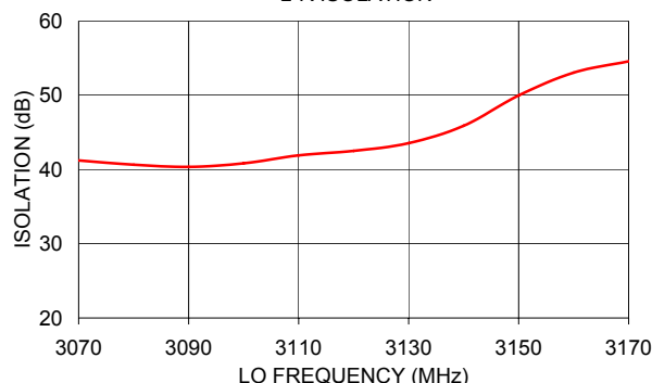
MCA-36FLH+ L-R ISOLATION
