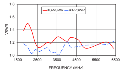
ZN8PD-642W-S+ VSWR
