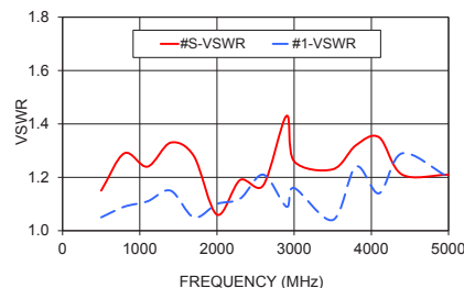
ZN8PD1-53-S+ VSWR
