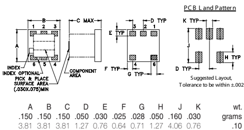
AT790 (SBTC-2-20+)
