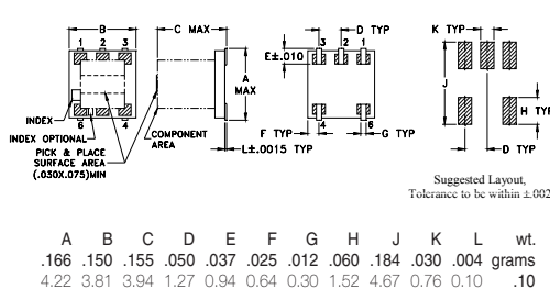
AT1029 (SBTC-2-20L+)
