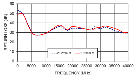
086-6KM+ RETURN LOSS
